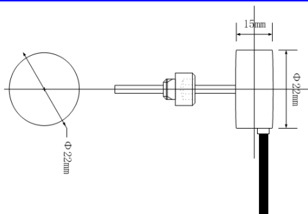
HSW1207——手持式
