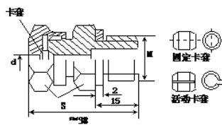
卡套螺纹示意图
