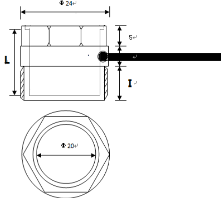
HSW1205——无固定装置、直插式
