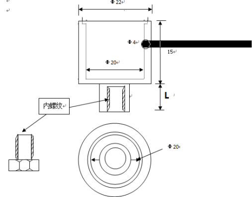
HSW1204B——表面安装式
